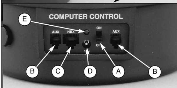
Fig. 2 (inserto): Panel de Control. (A) interruptor general; (B); puertos auxiliares; (C)puerto de controlador (HBX); (D) conector 12 Vcc; (E) LED - luz indicadora de corriente.
