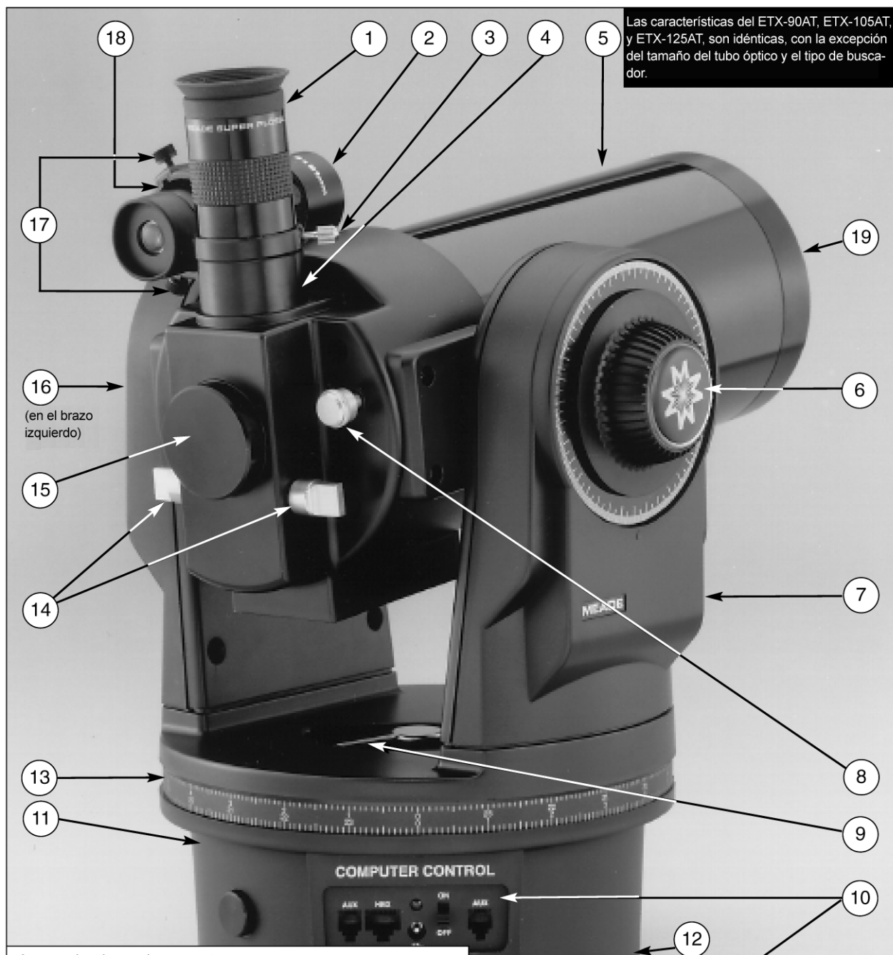
Fig. 1: El Telescopio ETX-90AT
